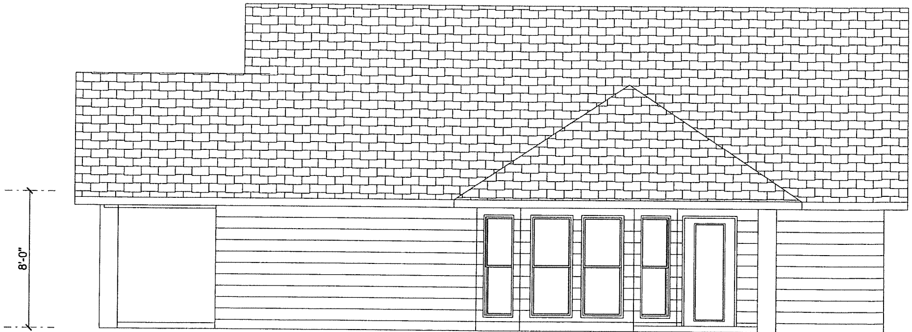
RIGHT ELEVATION
